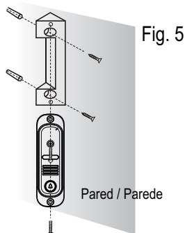
Instalación con Adaptador de Ángulo Instalação do Adaptador de ângulo
